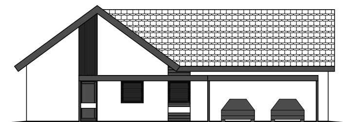
pohled přední
